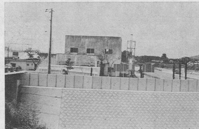
完成した水防壁（共同し尿処理場）
