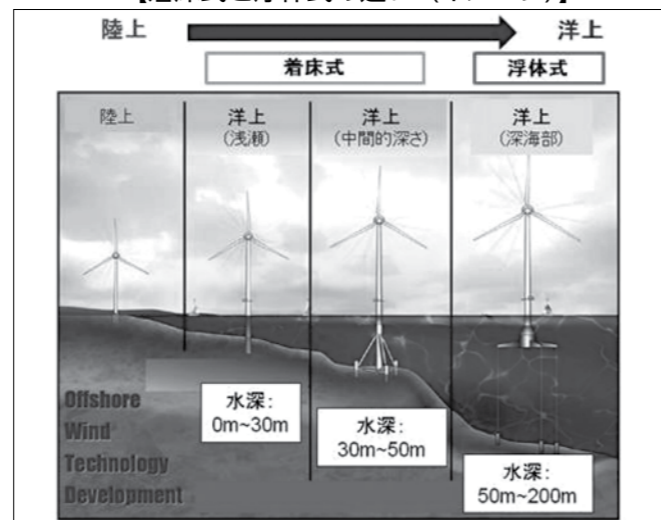
【着床式と浮体式の違い (イメージ)】
