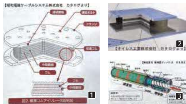
1 積層ゴム支承 2 弾性すべり支承 3 減衰コマ型ダンパー
