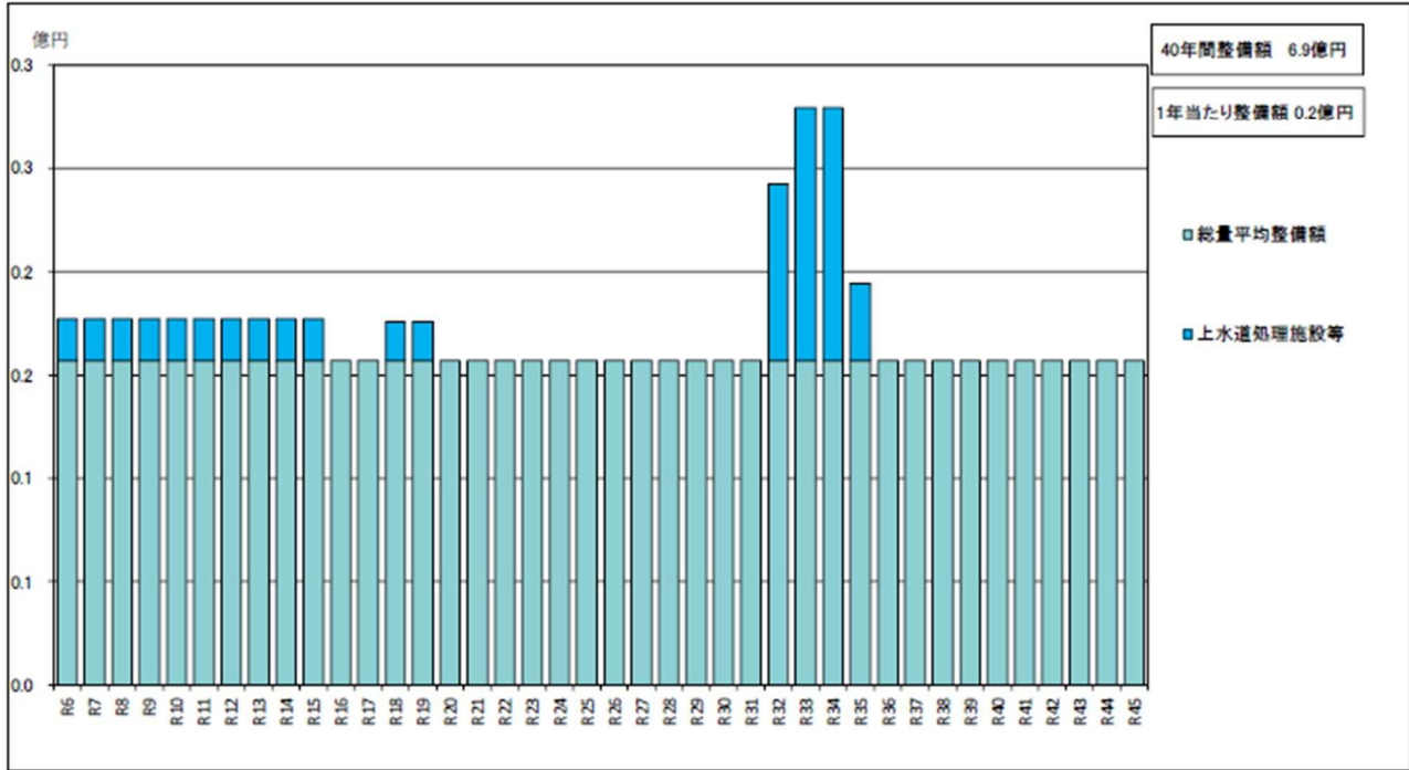
図 4-1-6 工業用水道の更新費用の試算結果
