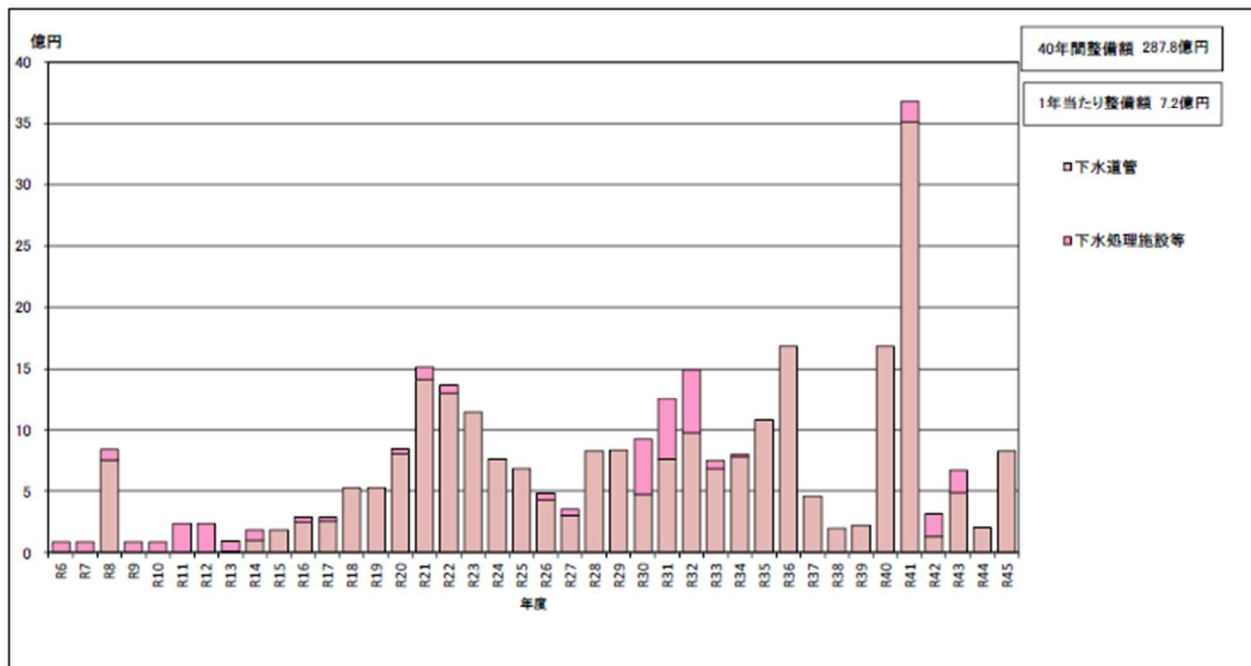
図 4-1-5 下水道施設の更新費用の試算結果
