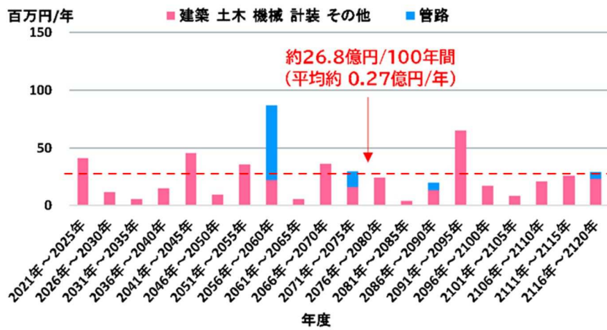
図 4-1-12 設定耐用年数で更新した場合の将来の更新費用
