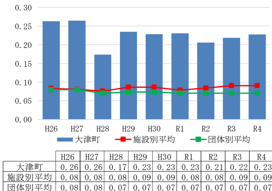
図 2-4-14 導送配水管使用効率
